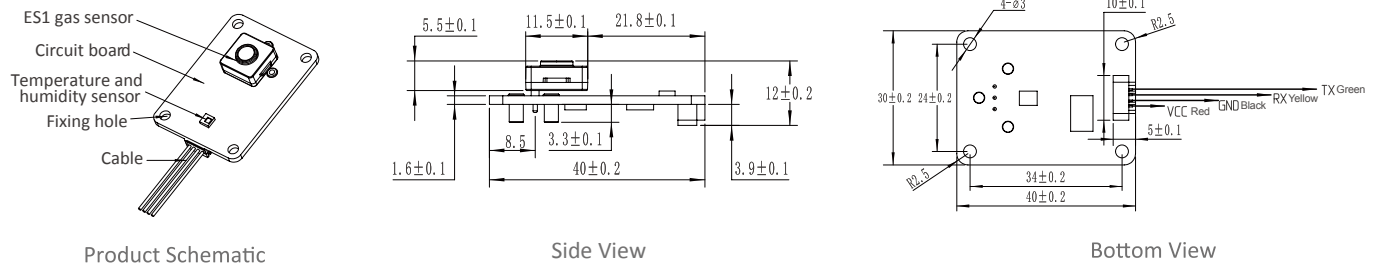
TB200B-ES1-ClO 2 Dimension diagram
